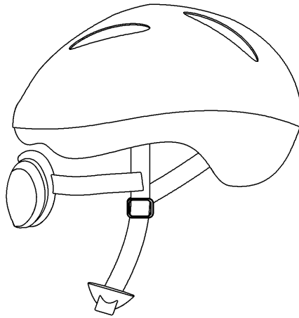
우측면도
